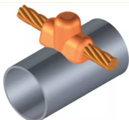
CABLE PASANTE HORIZONTAL SOBRE TUBO PERPENDICULAR
